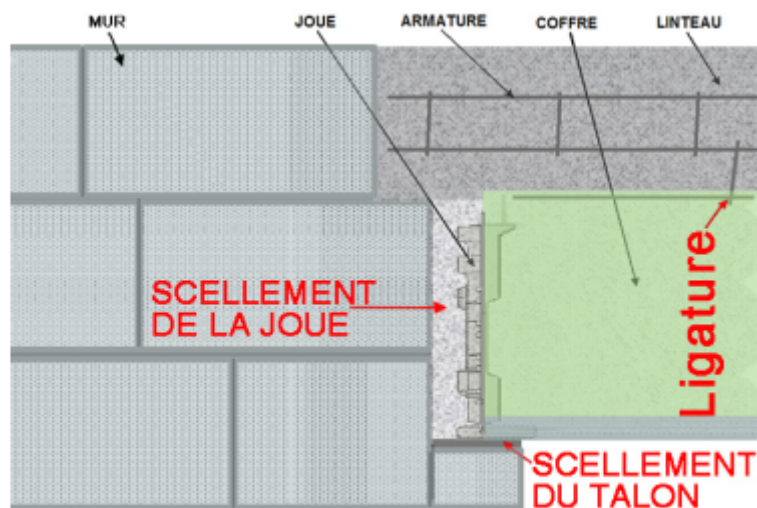
COUPE TRANSVERSALE DU COFFRE ET DE LA JOUE EN SITUATION DANS LE MUR.
