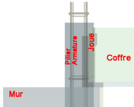
Pose en maçonnerie sismique = passage du pilier dans la joue, vue de face, côté extérieur
