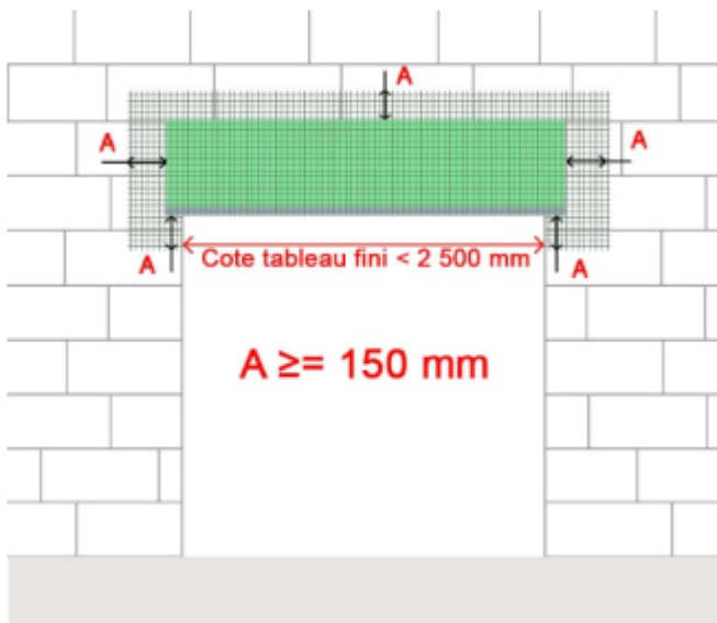
Renforcement de l'enduit jusqu'à 2500 mm
