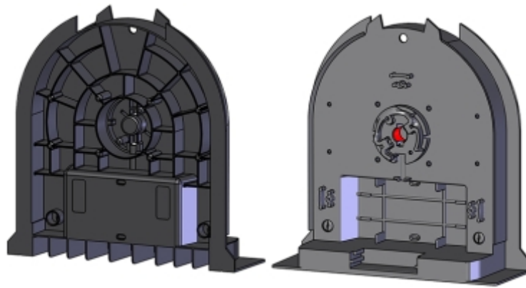
V.6 – Joue PS T 280/300
