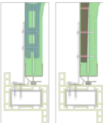
Rail PVC à languette + renfort
