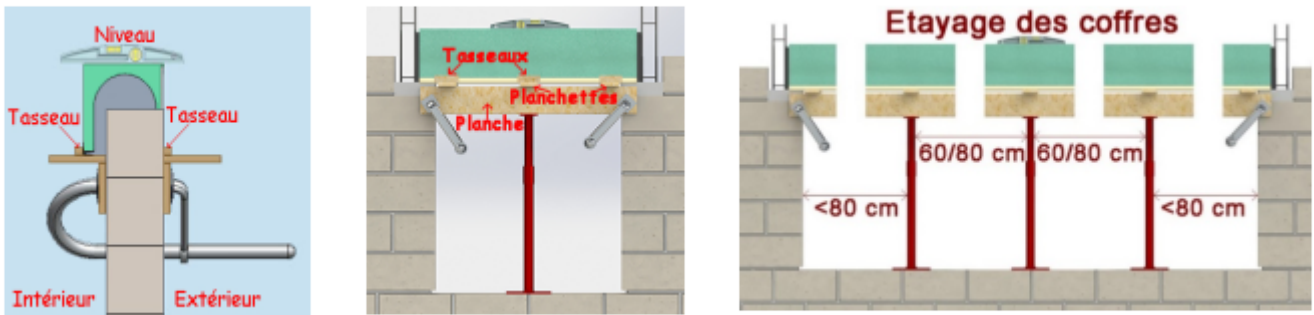
Blocage des jambage, Mise à niveau horizontal et vertical, Eaiement du coffre et maintien de la planéité.
