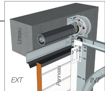
Vue extérieure Joint avec 2 lèvres
