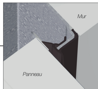
Joint à lèvres (sur rails verticaux)
