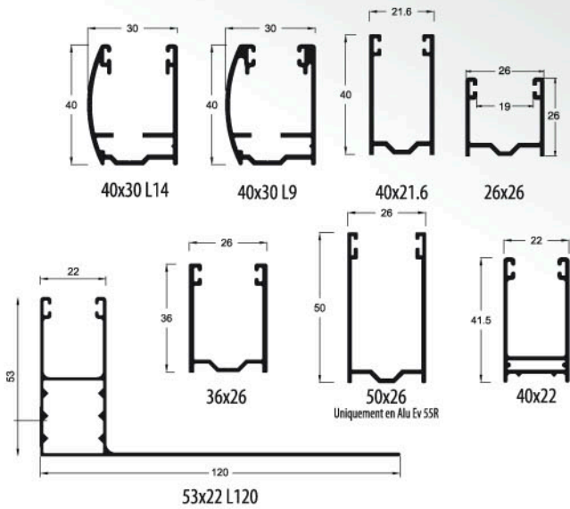
Coffres tunnel et volet Tradi
