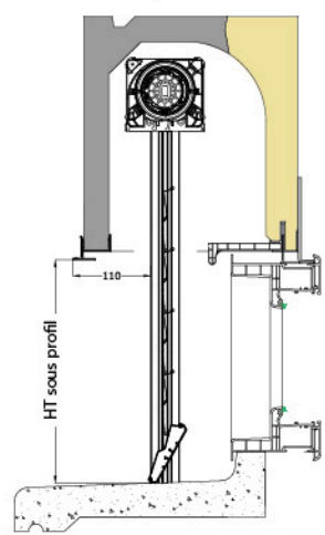
BSO en position fermée
