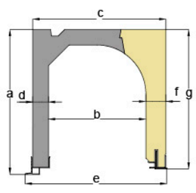
BSO en position fermée
