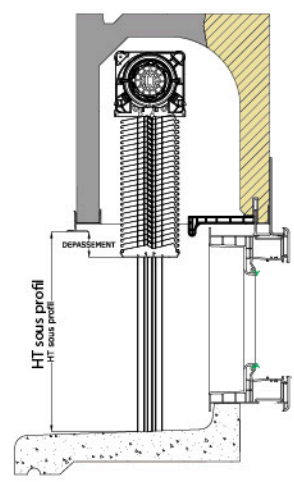
BSO en position ouverte Disposition 68-4 uniquement
